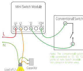
Diagram 1: For 1 Gang Mini Module
