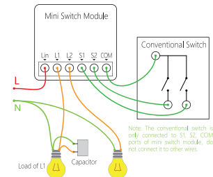
Diagram 2: For 2 Gang Mini Module
